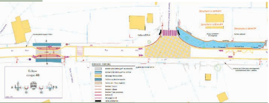
Schéma des futurs travaux de sécurisation de la rue Armor
